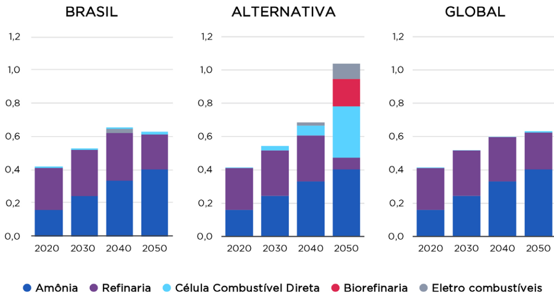
GRÁFICO 25 USOS DIRETOS DO HIDROGÊNIO (EM Mt)
